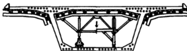
Рисунок 5 - Установка щита внутренней съёмной опалубки второй очереди бетонирования
