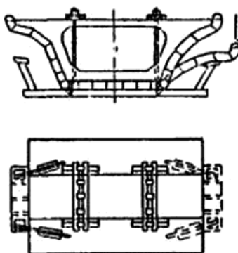
Рисунок 6 - Распалубливание подвесной опалубки
