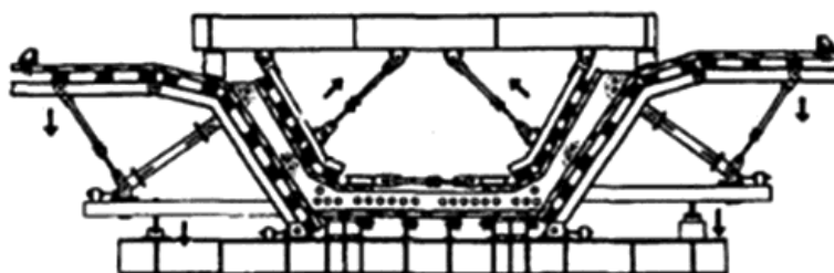
Рисунок 4 - Установка щита внутренней съемной опалубки первой очереди бетонирования
