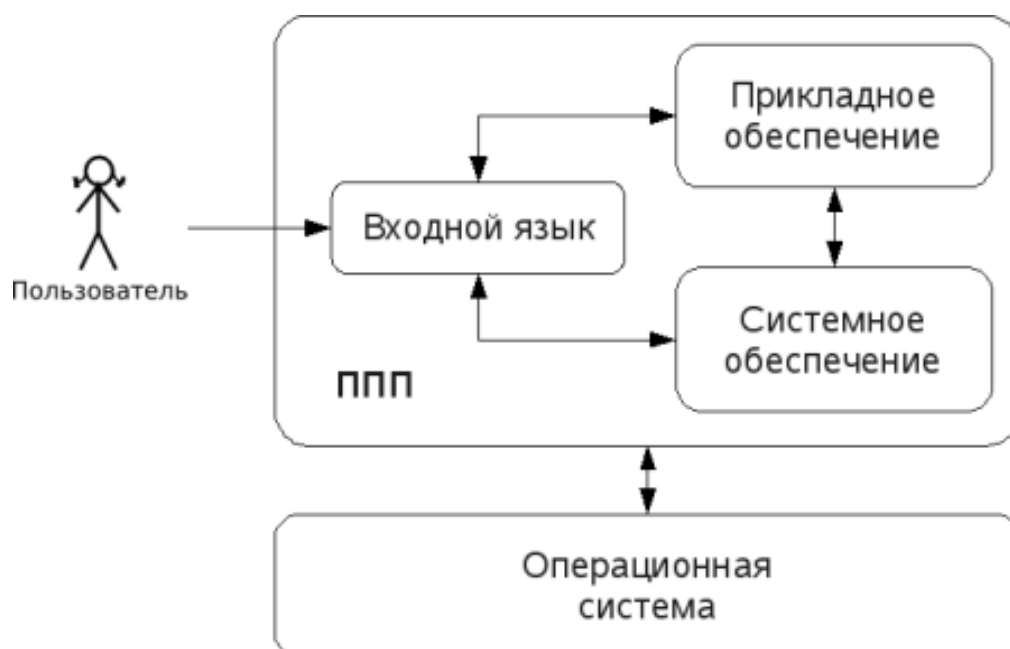
Рис. 2. Структура ППП.
